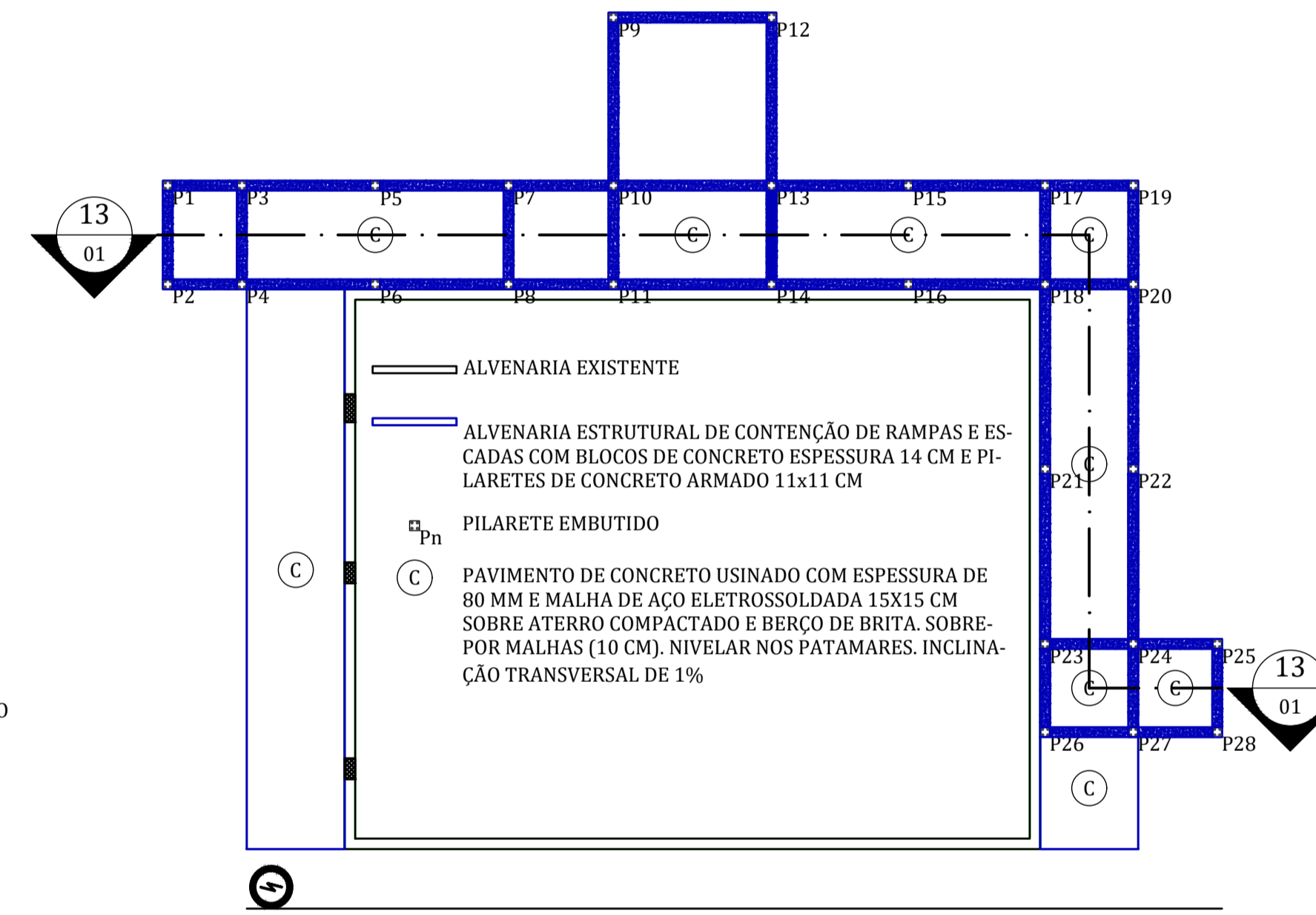
13 EDIFÍCIO H - MUROS DE CONTENÇÃO DE RAMPAS E ESCADAS ESCALA 1:80
