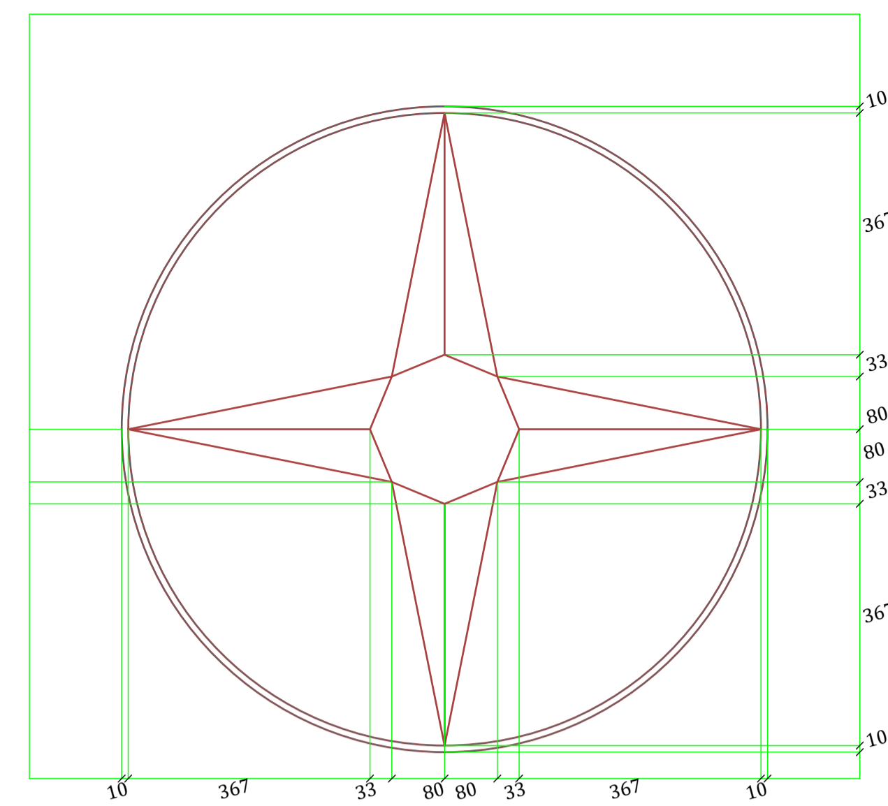
28 GABARITO PONTOS CARDEAIS ESCALA 1:80
