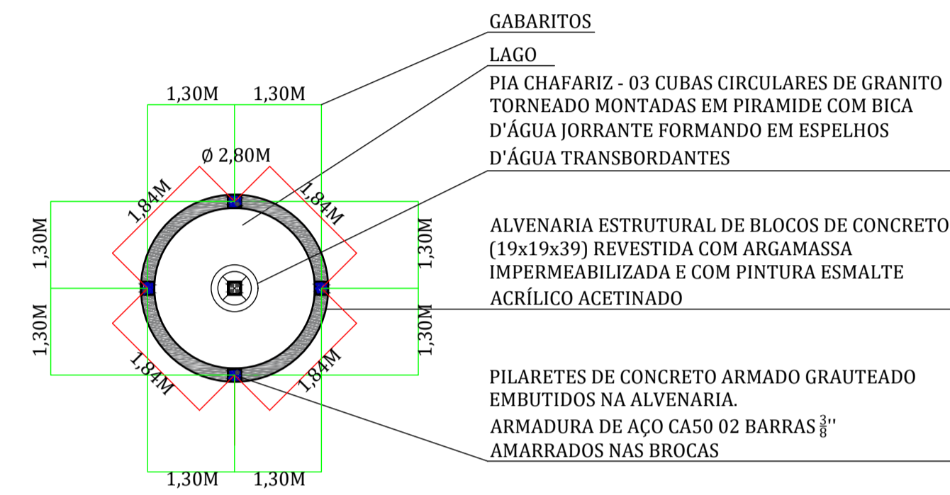
25 PLANTA DE ALVENARIA EMBASAMENTO DO CHAFARIZ ESCALA 1:80
