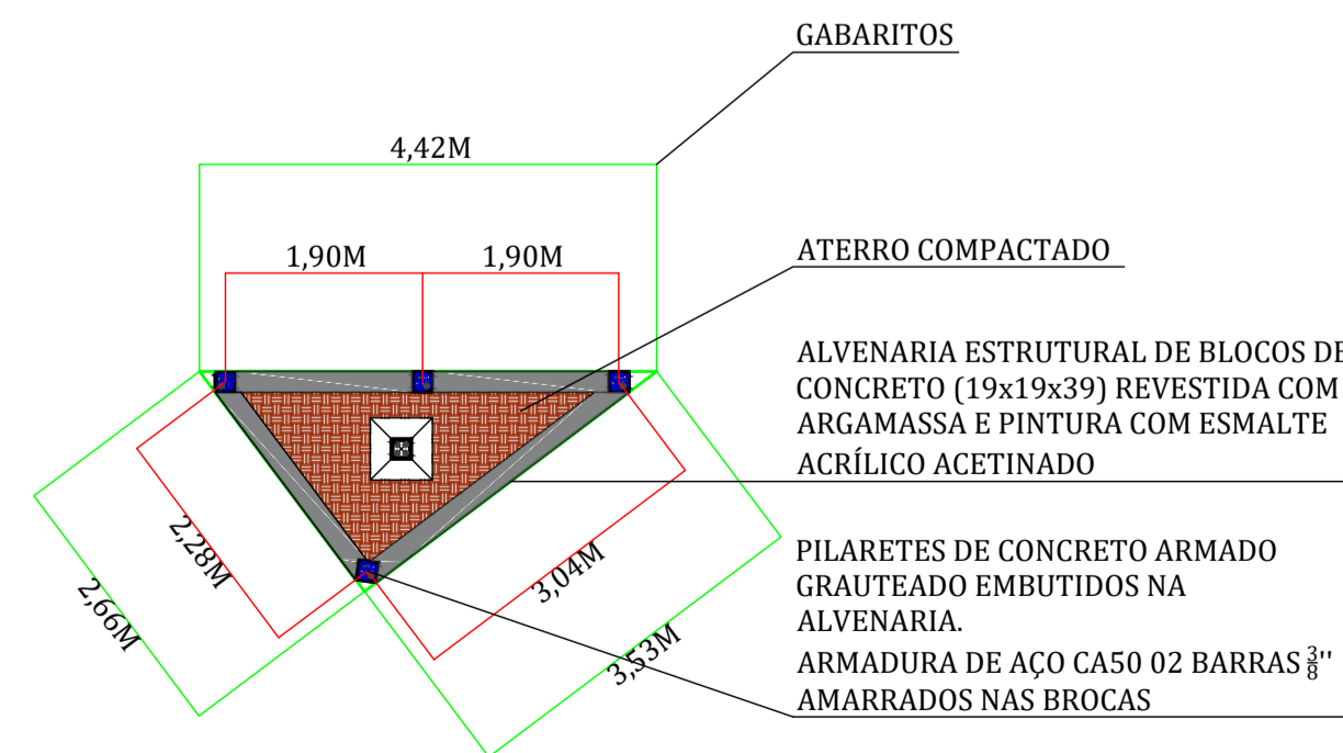
19 PLANTA DE ALVENARIA EMBASAMENTO DA ESCULTURA ESCALA 1:80
