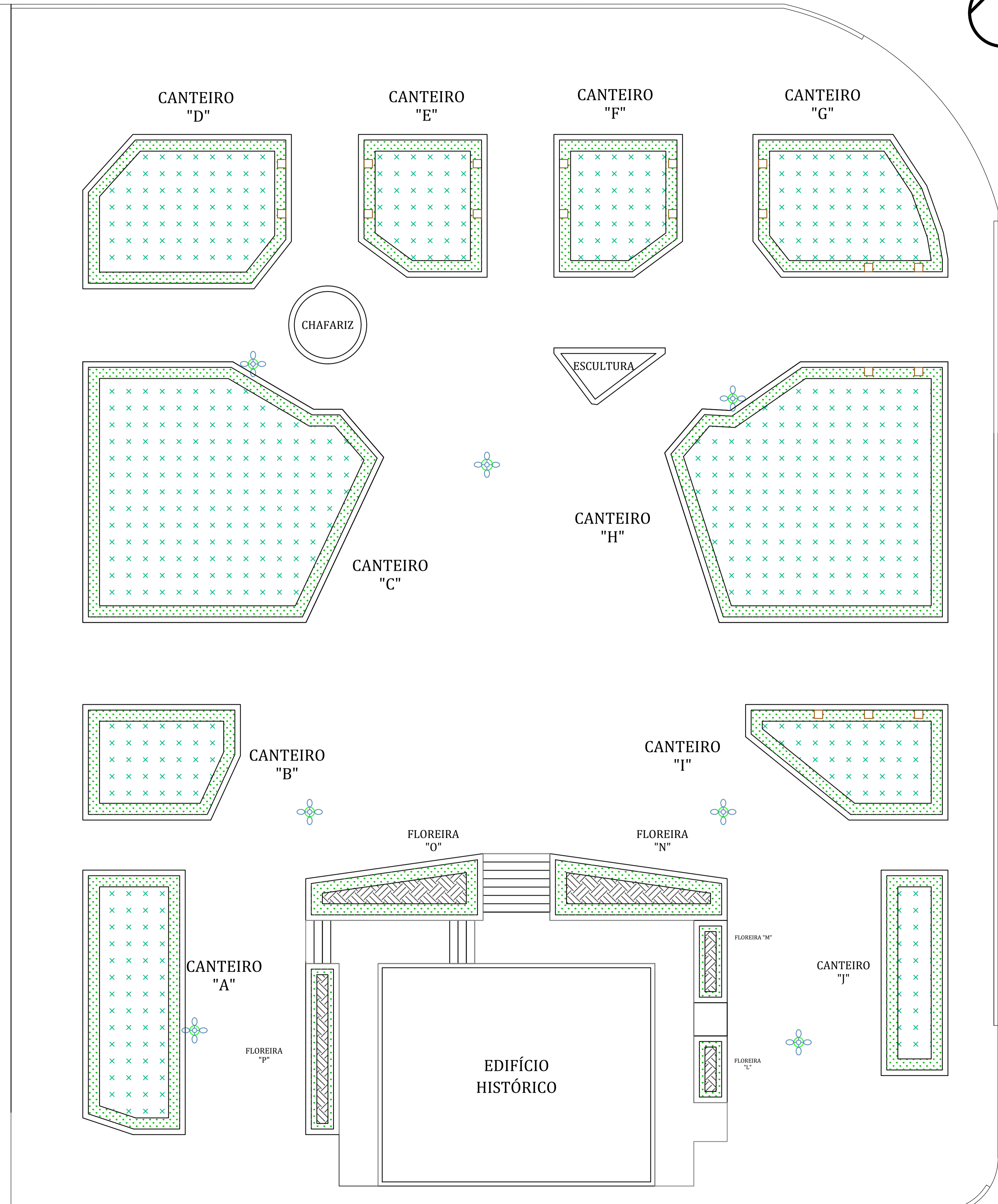
36 PLANTA DE REVITALIZAÇÃO PAISAGÍSTICA ESCALA 1:80
