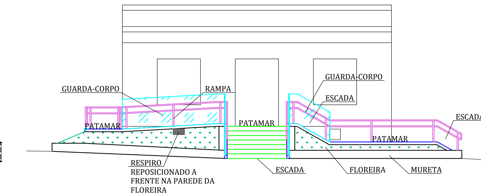
09 EDIFÍCIO H - ELEVÇÃO SITUAÇÃO FUTURA ESCALA 1:80
