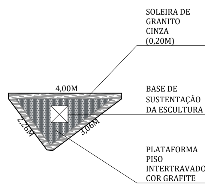
18 PLANTA EMBASAMENTO DA ESCULTURA ESCALA 1:80
