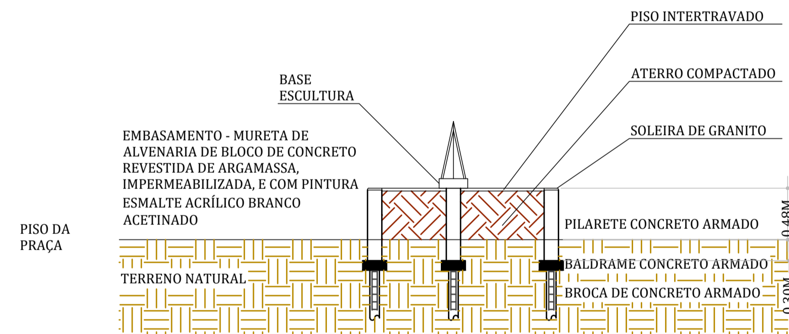
22 CORTE ESQUEMÁTICO EMBASAMENTO DA ESCULTURA ESCALA 1:80
