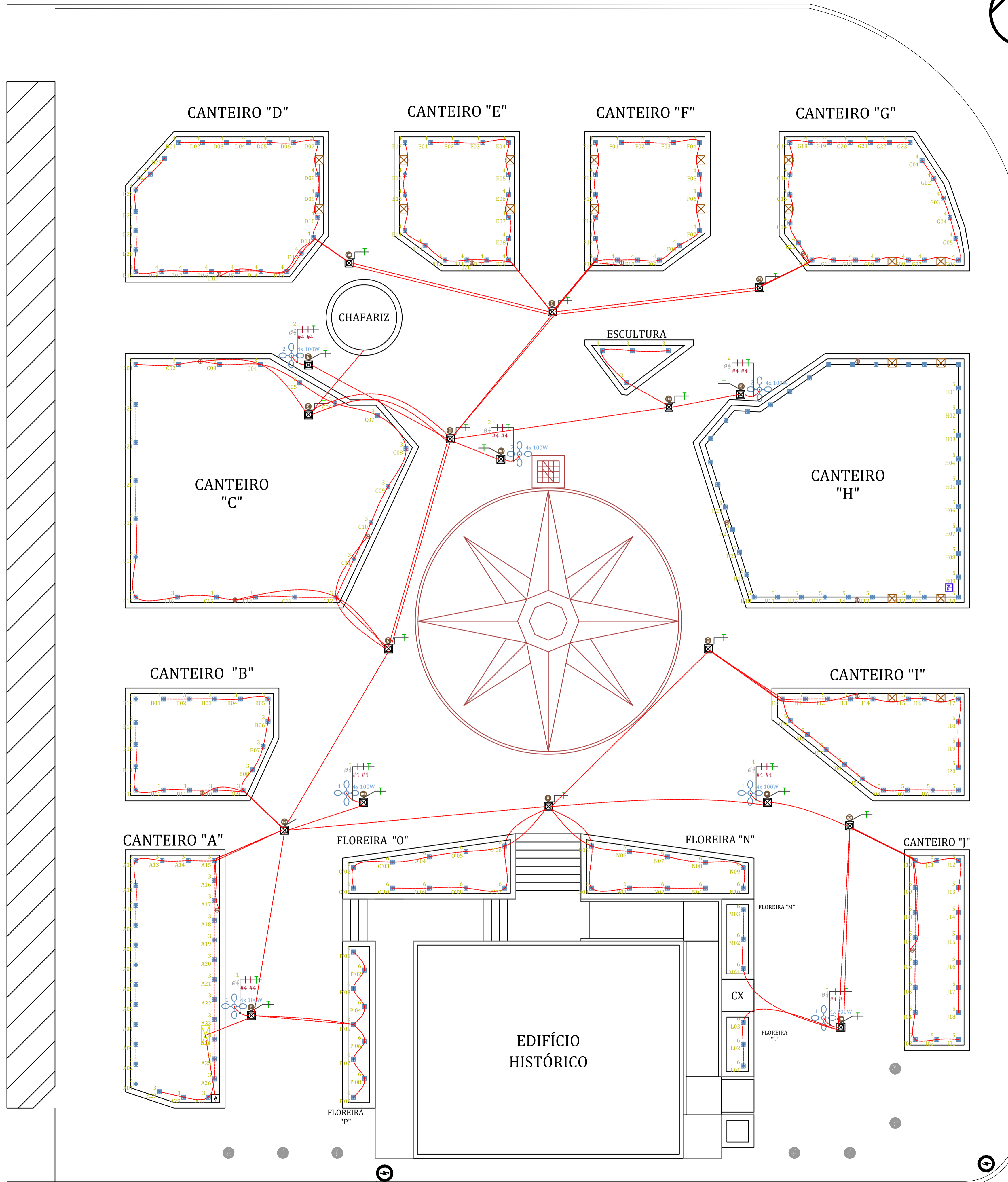
38 PLANTA DE INSTALAÇÕES ELÉTRICAS E ILUMINAÇÃO ESCALA 1:80
