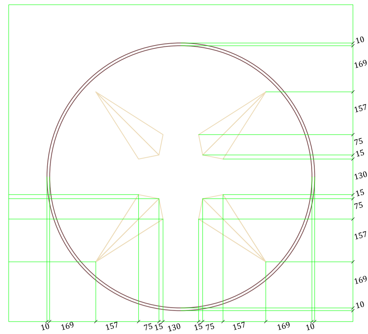
29 GABARITO PONTOS COLATERAIS ESCALA 1:80
