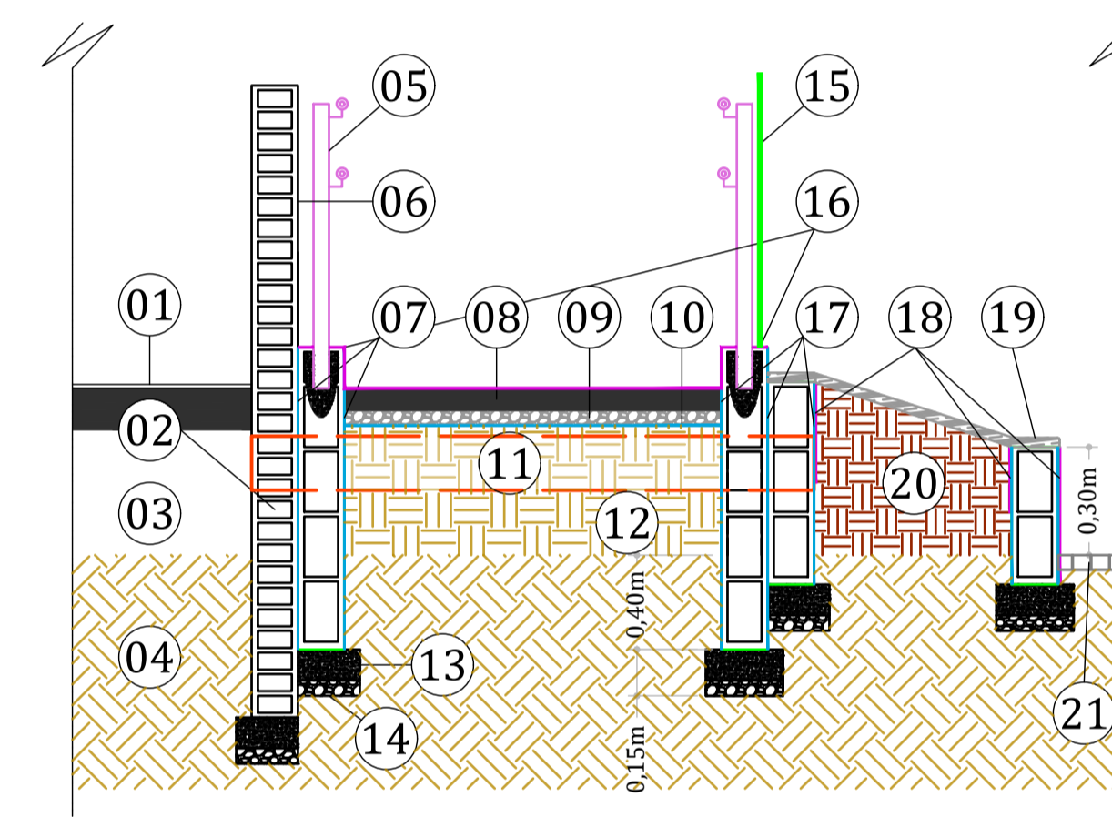
15 CORTE LONGITUDINAL RAMPA - MURO DE CONTENÇÃO RAMPAS E ESCADAS ESCALA 1:80
