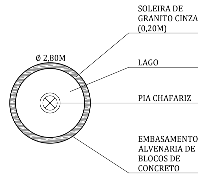
24 PLANTA EMBASAMENTO DO CHAFARIZ ESCALA 1:80
