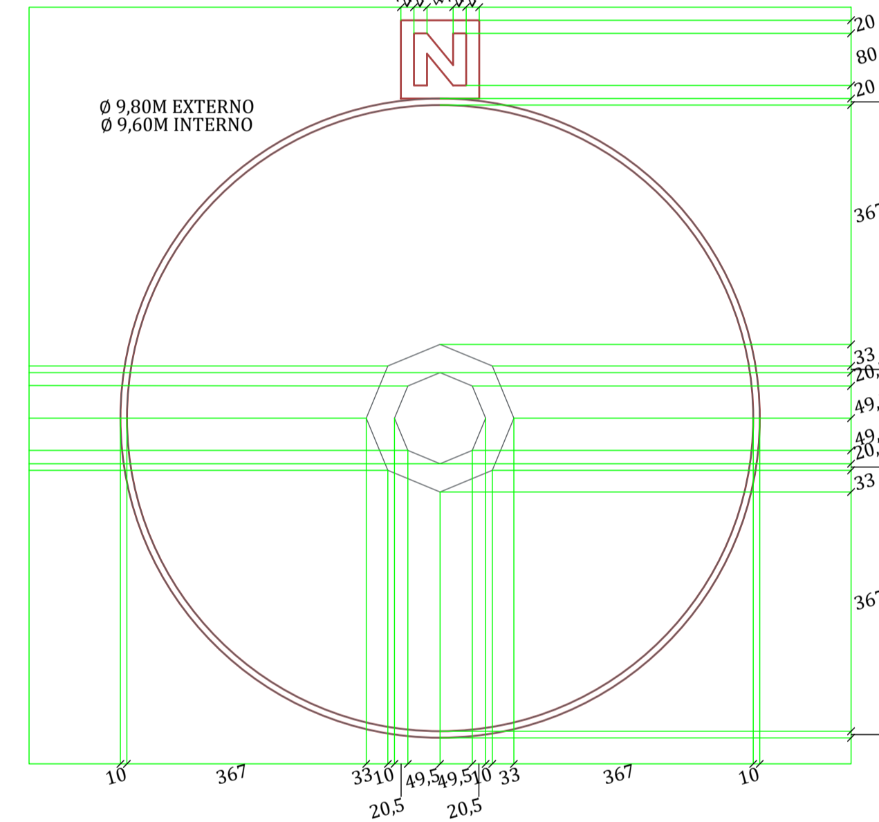
23 GABARITO ANEL CIRCUDANTE, OCTÓGONO, ORLA E LETRA "N" ESCALA 1:80
