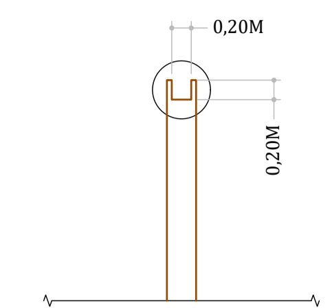
35 PILAR - VISTA LATERAL - DETALHE SAMBLADURA SEM ESCALA
