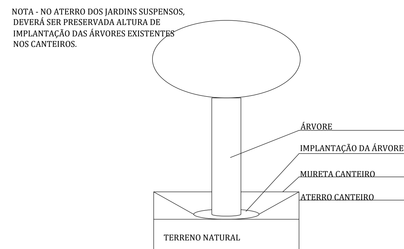
37 DETALHE DE ELEVÇÃO DO JARDIM SEM ESCALA
