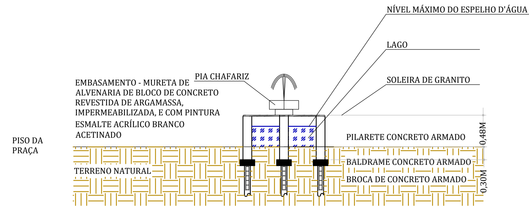
27 CORTE ESQUEMÁTICO EMBASAMENTO DO CHAFARIZ ESCALA 1:80
