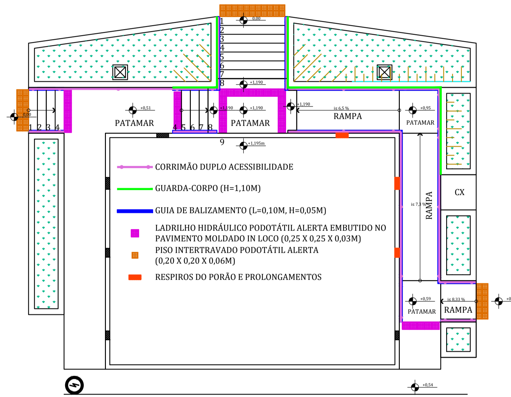
11 EDIFÍCIO H - SITUAÇÃO FUTURA - COTAS E ACESSIBILIDADE ESCALA 1:80
