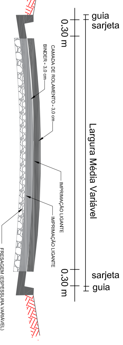
Corte Transversal Esquemático Sem escala
