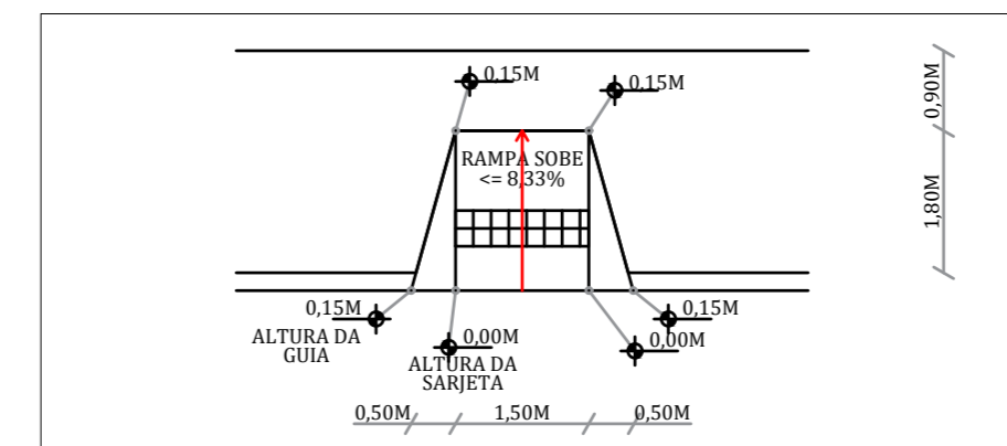
DETALHE GÊNÉRICO - RAMPAS ACESSIBILIDADE - NBR 9050:2020 SEM ESCALA
