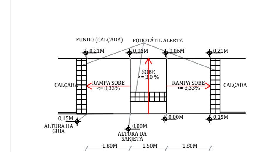
DETALHE GÊNÉRICO - CALÇADA REBAIXADA - NBR 9050:2020 SEM ESCALA
