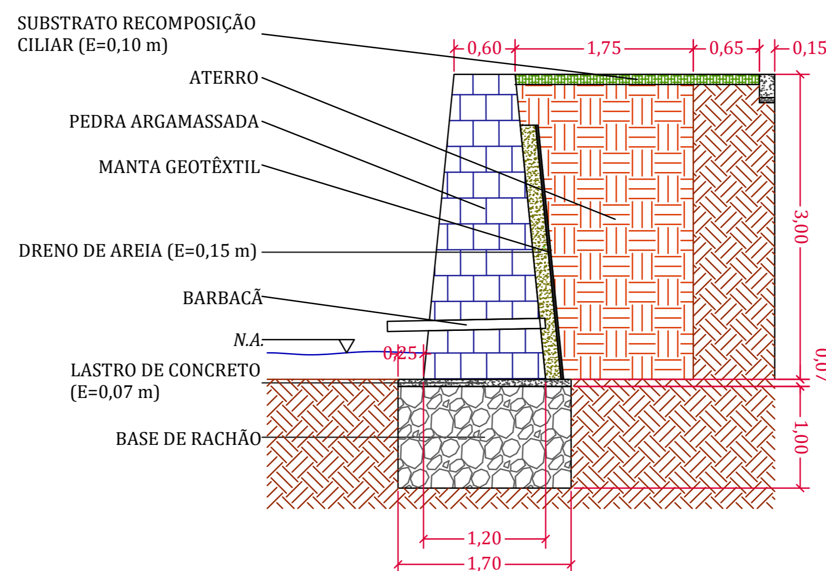
05 DETALHE CONSTRUTIVO SEM ESCALA
